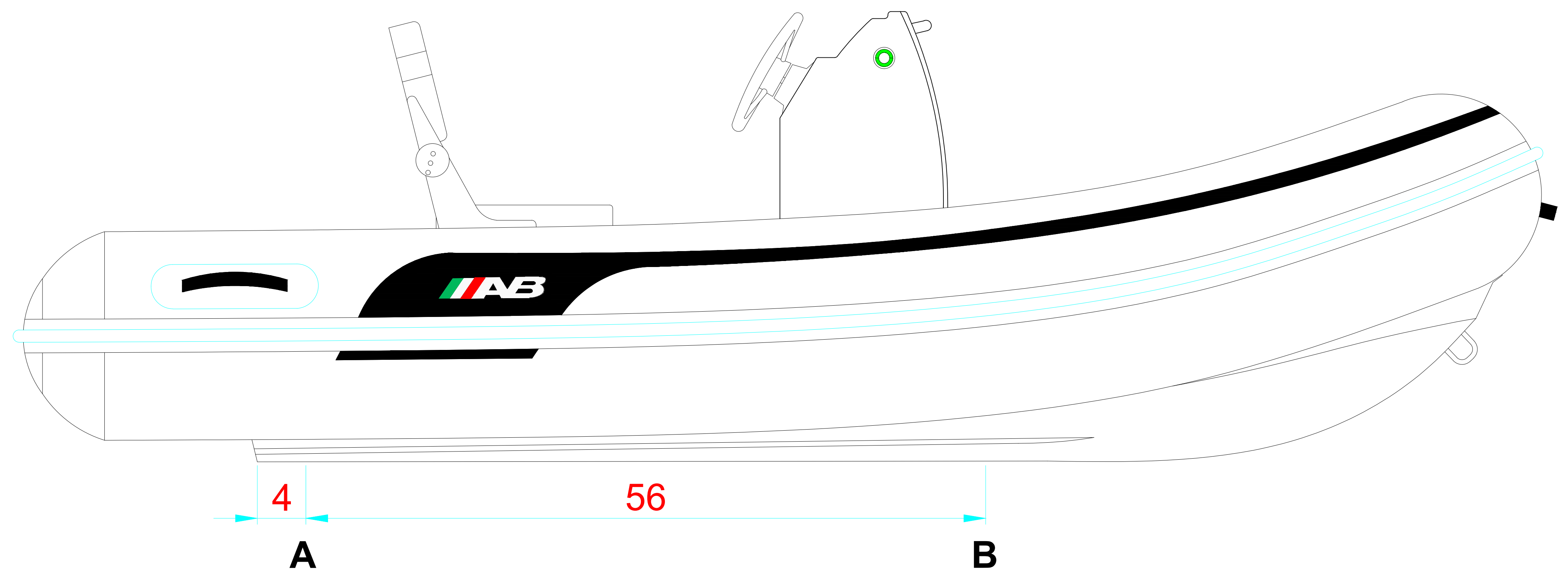
LONGITUDINAL PROFILE VISTA LATERAL
