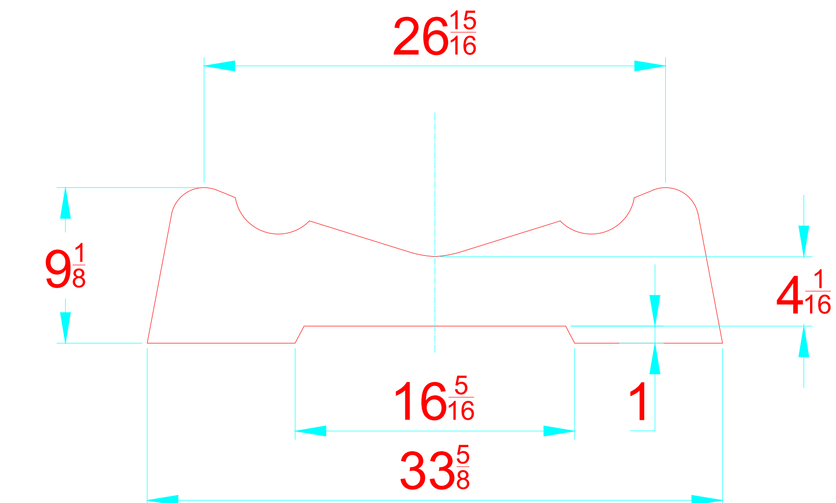
TRANSVERSAL SECTION "B" SECCION TRANSVERSAL "B"
