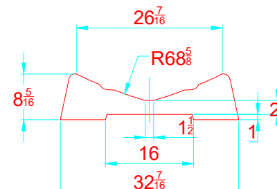
TRANSVERSAL SECTION "B" SECCION TRANSVERSAL "B"
