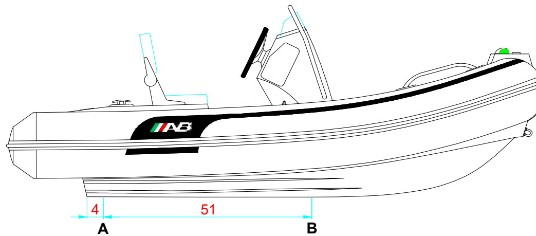
LONGITUDINAL PROFILE VISTA LATERAL
