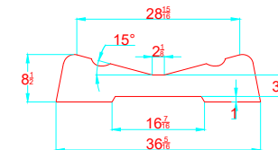
TRANSVERSAL SECTION "B" SECCION TRANSVERSAL "B"
