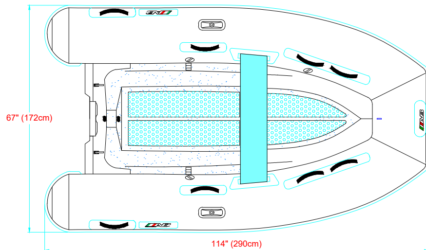
PLANT VIEW VISTA EN PLANTA
