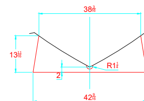
TRANSVERSAL SECTION "B" SECCION TRANSVERSAL "B"
